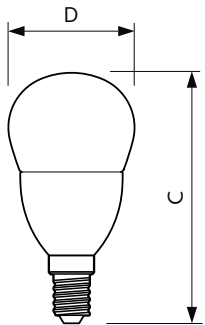
MASTER LEDlustre DT 5.5-40W E14 P48 CL
